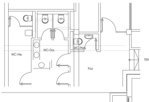
KG / WC
